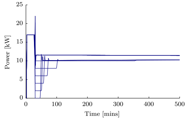
(d) Power Consumption, P_0 = 17 \text{ kW}
