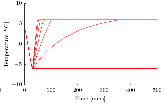
(d) Temperature, P_0 = 17 \text{ kW}
